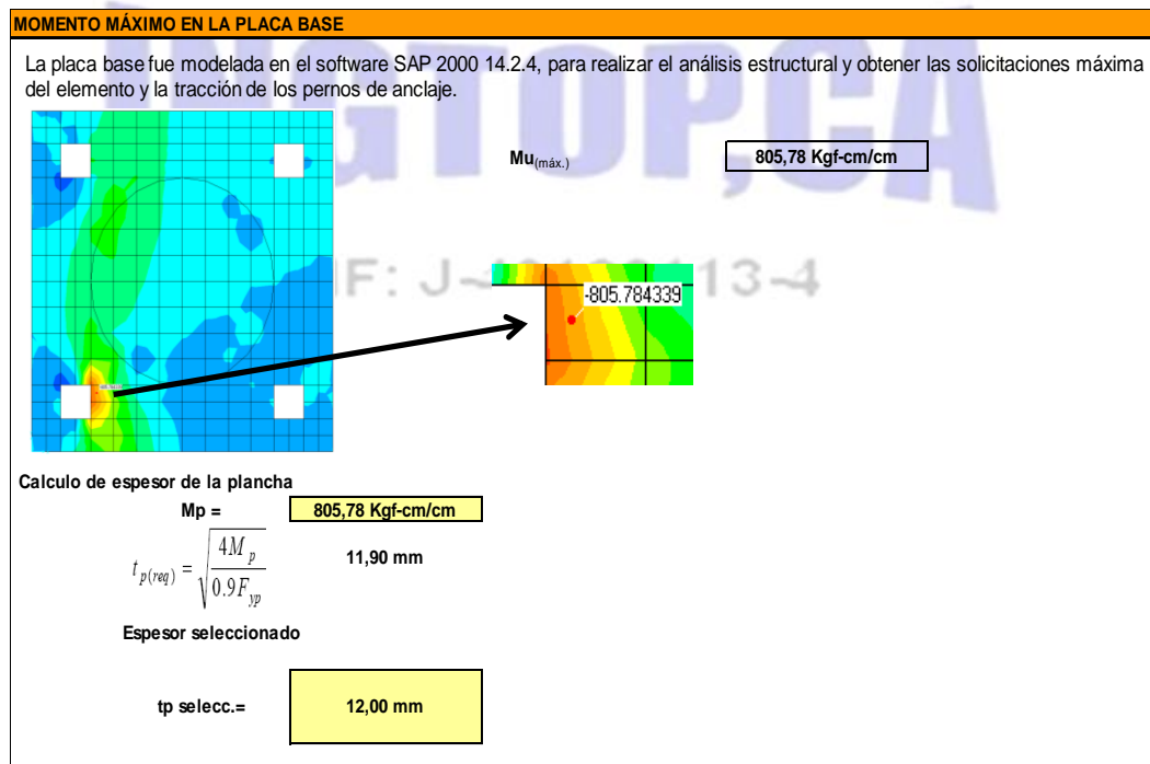
Figura 12.2.1: Hoja de cálculo – Diseño de espesor de placa base.
